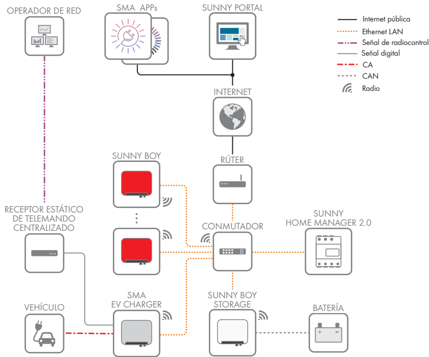
Imagen 5: Estructura de la comunicación de la planta
