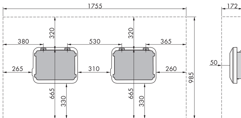
Imagen 8: Distancias recomendadas (Medidas en mm)
