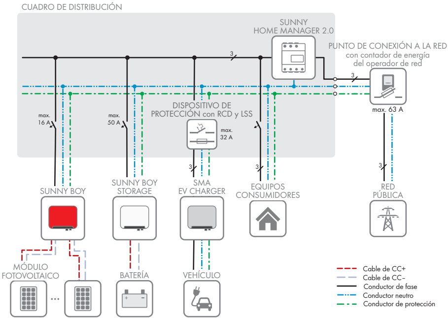
Imagen 4: Esquema de interconexión (ejemplo)
