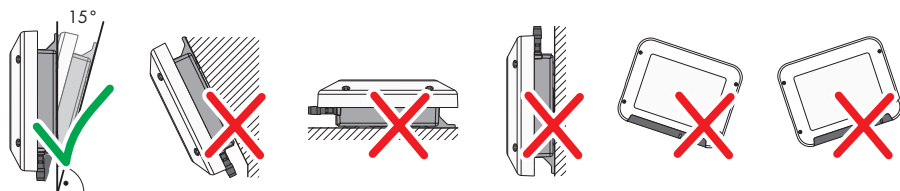
Imagen 6: Posiciones de montaje permitidas y no permitidas
