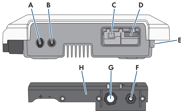
Imagen 9: Áreas de conexión y aberturas en la carcasa en la parte inferior del inversor
