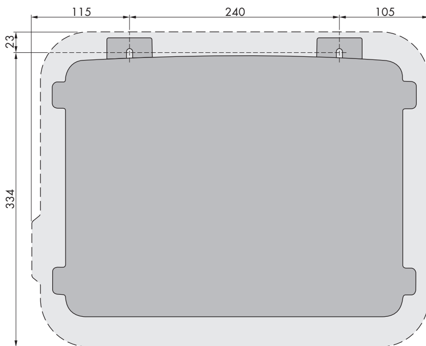
Imagen 7: Posición de los puntos de fijación (Medidas en mm)
